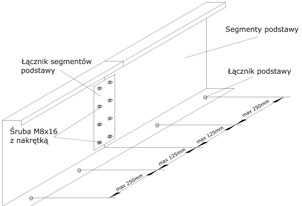
Rys. 3. Sposób łączenia segmentów podstaw pasm świetlnych
