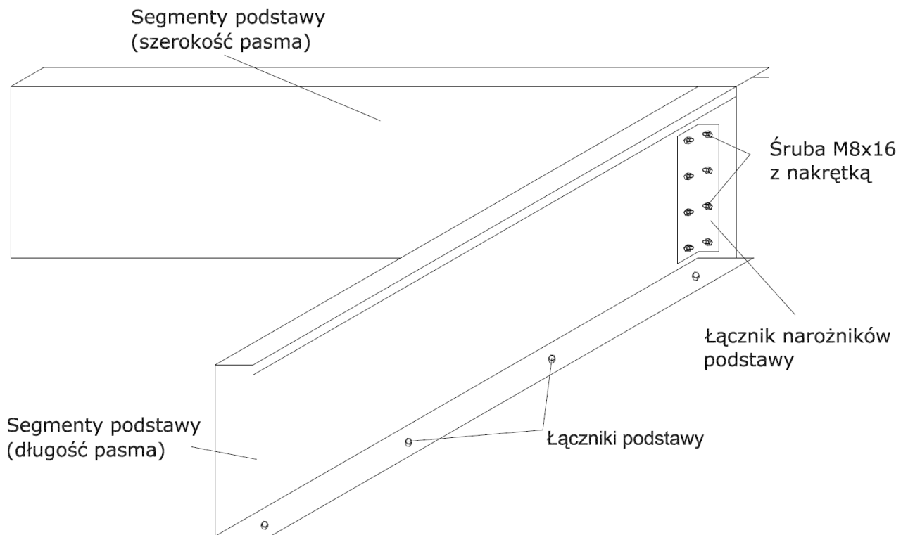
Rys. 4. Sposób łączenia narożników podstawy pasma świetlnego
