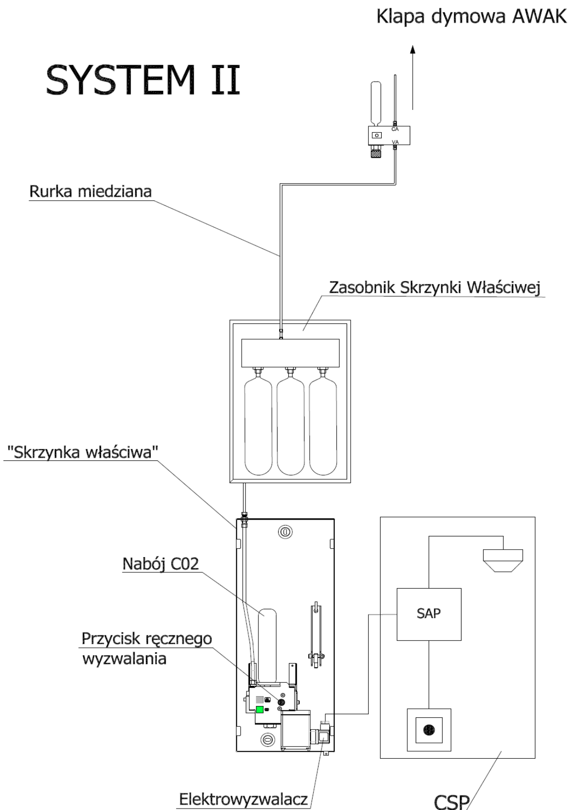
Rys.24.b. Sposób sterowania oddymianiem – System II
