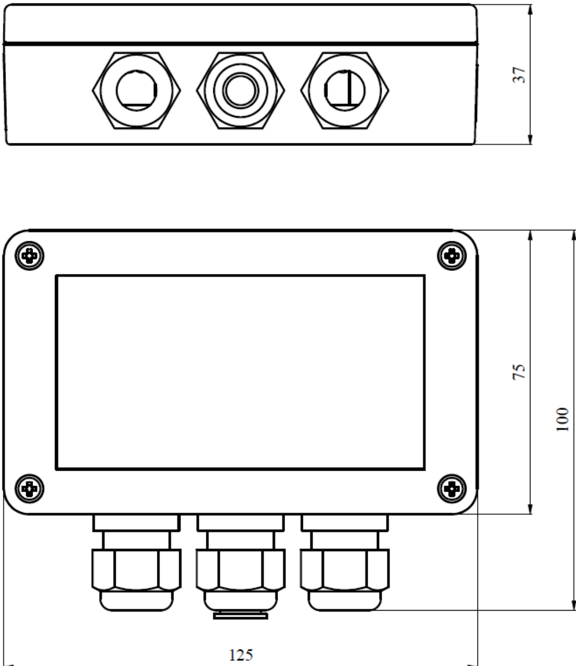
Rysunek 1 Wymiary zewnętrzne AKC-6000
