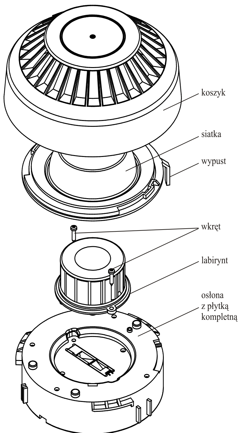
Rys. 8.1 Elementy czujki po demontażu
