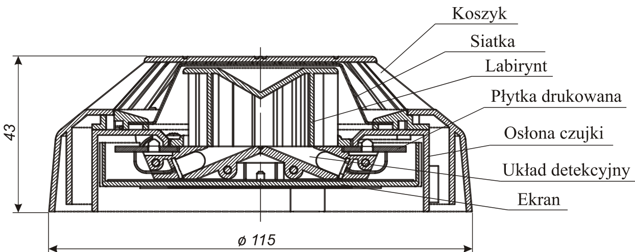
Rys. 6.1 Konstrukcja czujki DUR-40Ex
