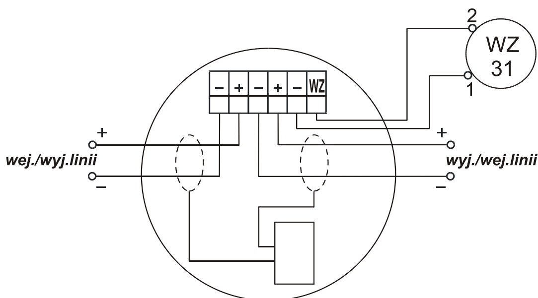
Rys 9.1. Zaciski gniazda współpracującego z wtykiem czujki
