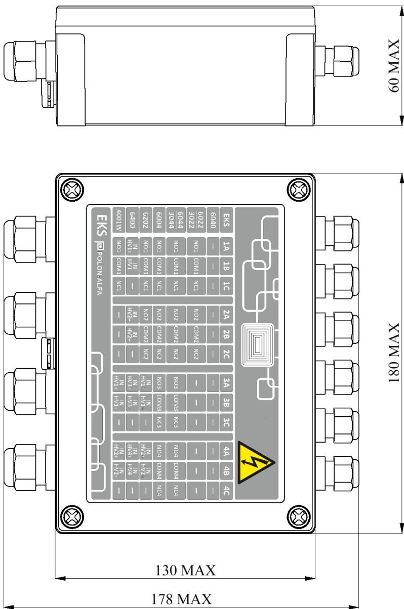
Rysunek 3.2 Wymiary EKS-3044
