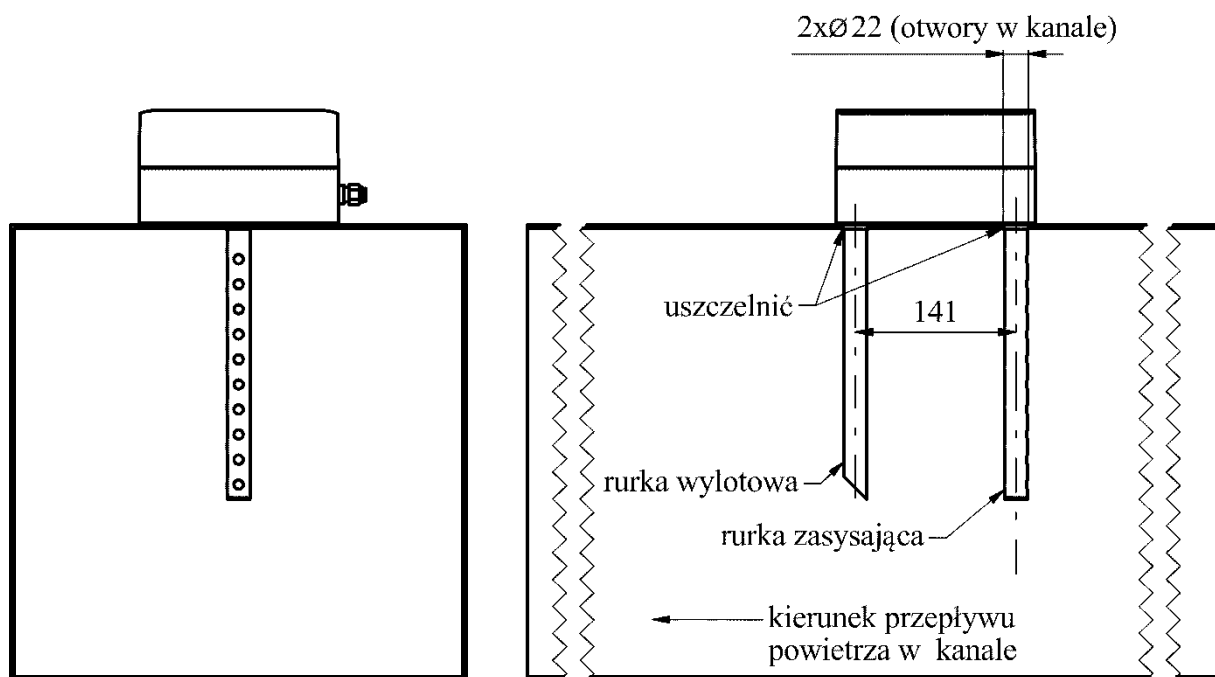
Rysunek 8.1 Przykład instalowania czujki DUO-6046K w kanale
