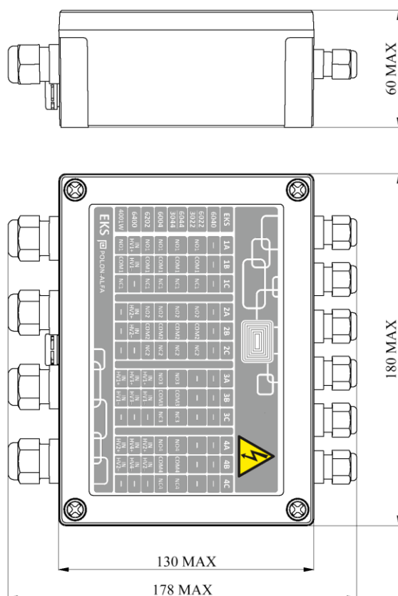
Rysunek 3.4 Wymiary EKS-6044
