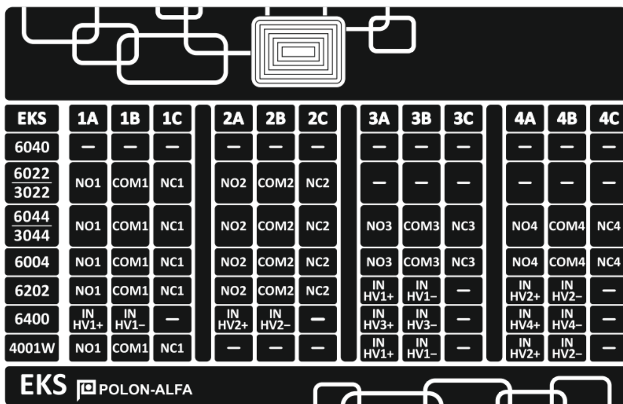
Rysunek 7.3 Pokrywa obudowy z funkcjami zacisków EKS-6000
