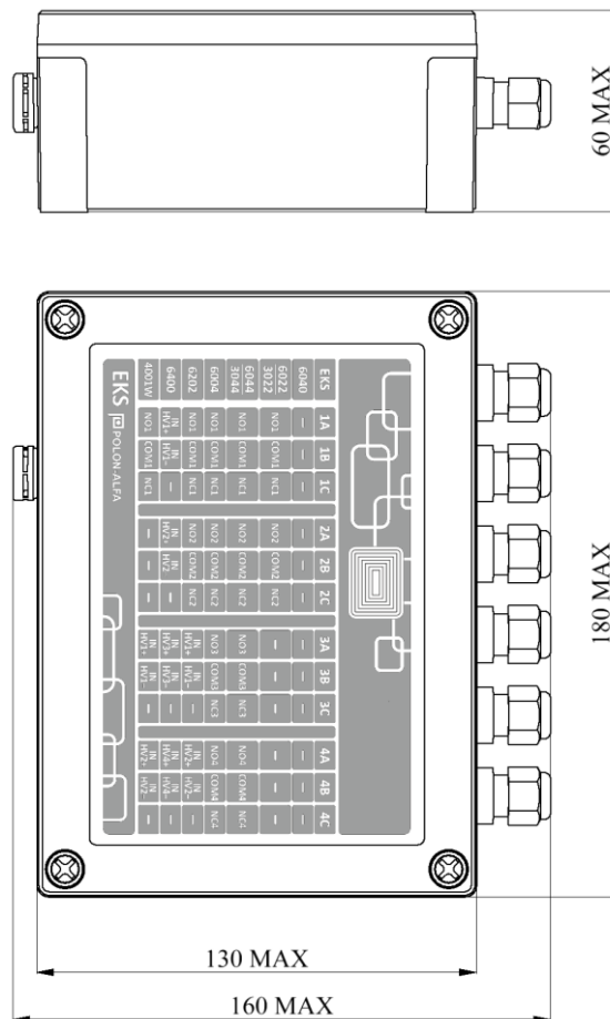
Rysunek 3.1 Wymiary EKS-6040
