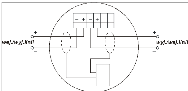
Rys 7.1 Zaciski gniazda współpracującego z wtykiem adaptera
