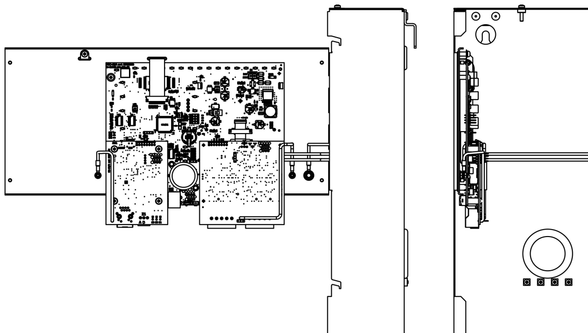
Rys. 5-3 Centrala z odchylonym panelem PSO-30
