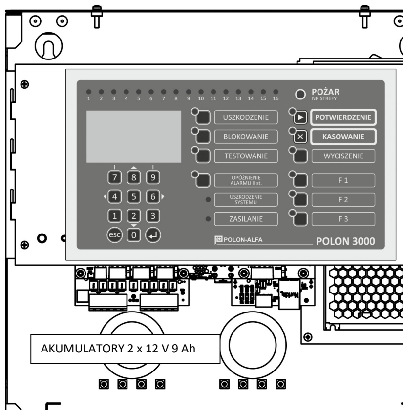
Rys. 6-2 Widok położenia akumulatorów w obudowie
