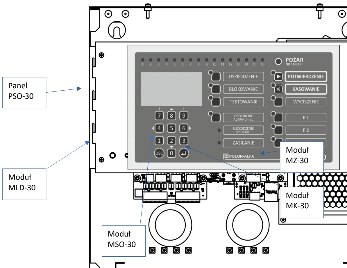
Rys. 5-2 Moduły centrali
