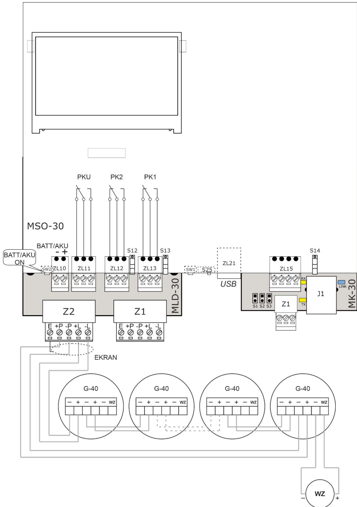
Rys. 5-8 Schemat podłączenia linii dozorowej pętlowej do modułu MLD-30
