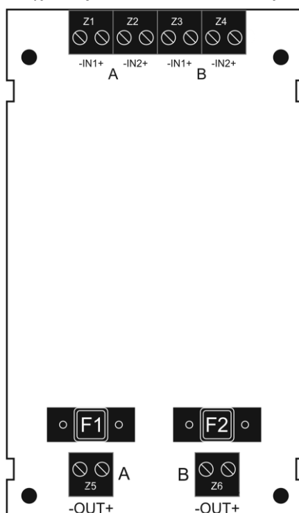
Rysunek 6.5.1. Opis wejść oraz wyjść złącz Modułu Redundancji Zasilania MRZ-60
