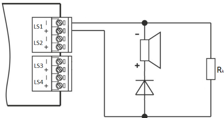
Rysunek 6.3.3. Przykład podłączenia sygnalizatora akustycznego do linii sygnałowej
