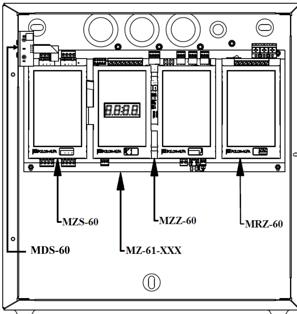
Rysunek 2.1.1. Rozmieszczenie modułów wewnątrz Pożarowego Zasilacza Buforowego
