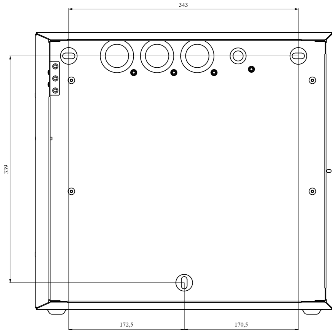
Rysunek 11.1.2. Wymiary montażowe obudowy M71
