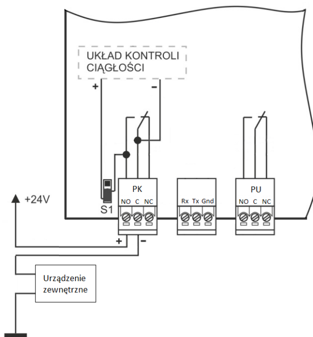
Rysunek 6.2.8.1. Rozmieszczenie styków przełącznika konfigurowalnego oraz przełącznika uszkodzenia
