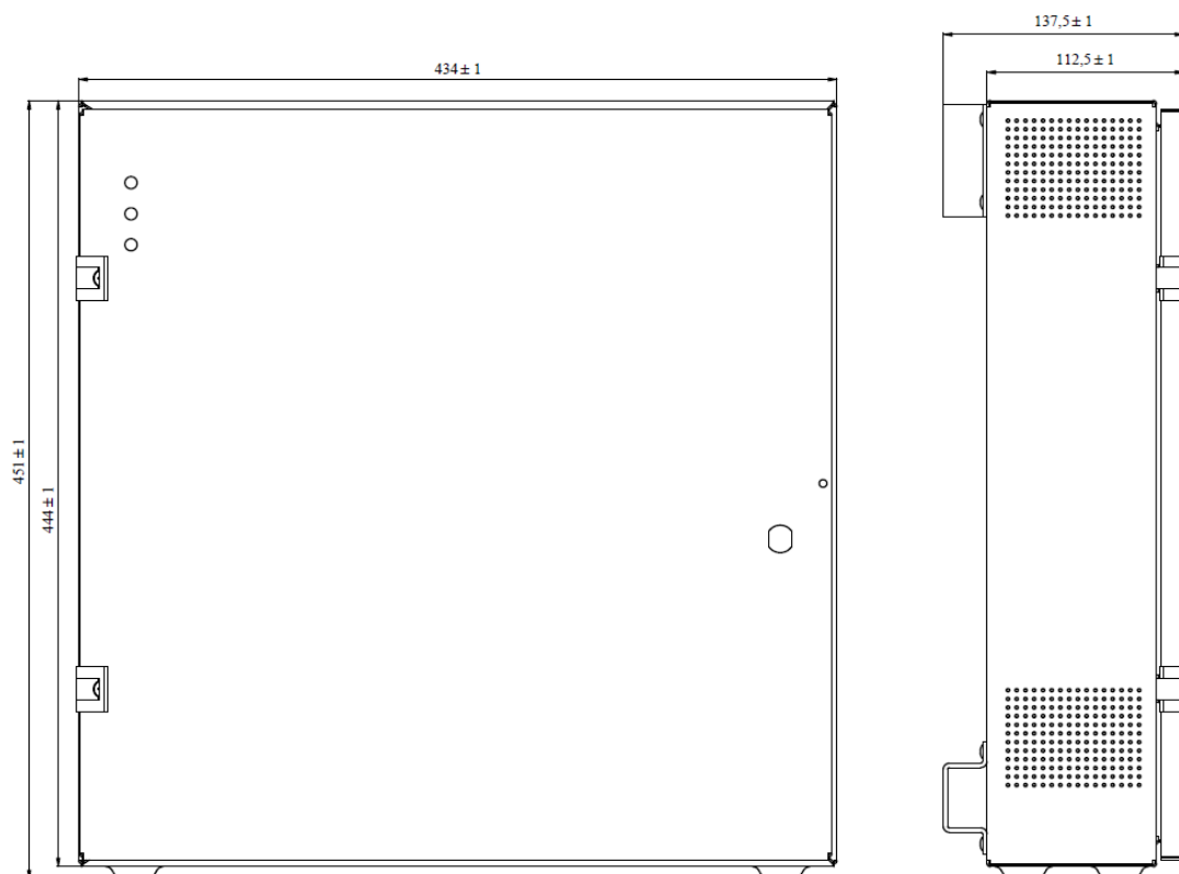
Rysunek 4.1. Obudowa M70
