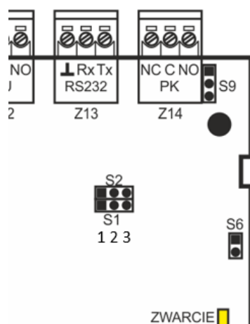
Rysunek 6.2.10.1. Numeracja złącza szpilkowego S1.
