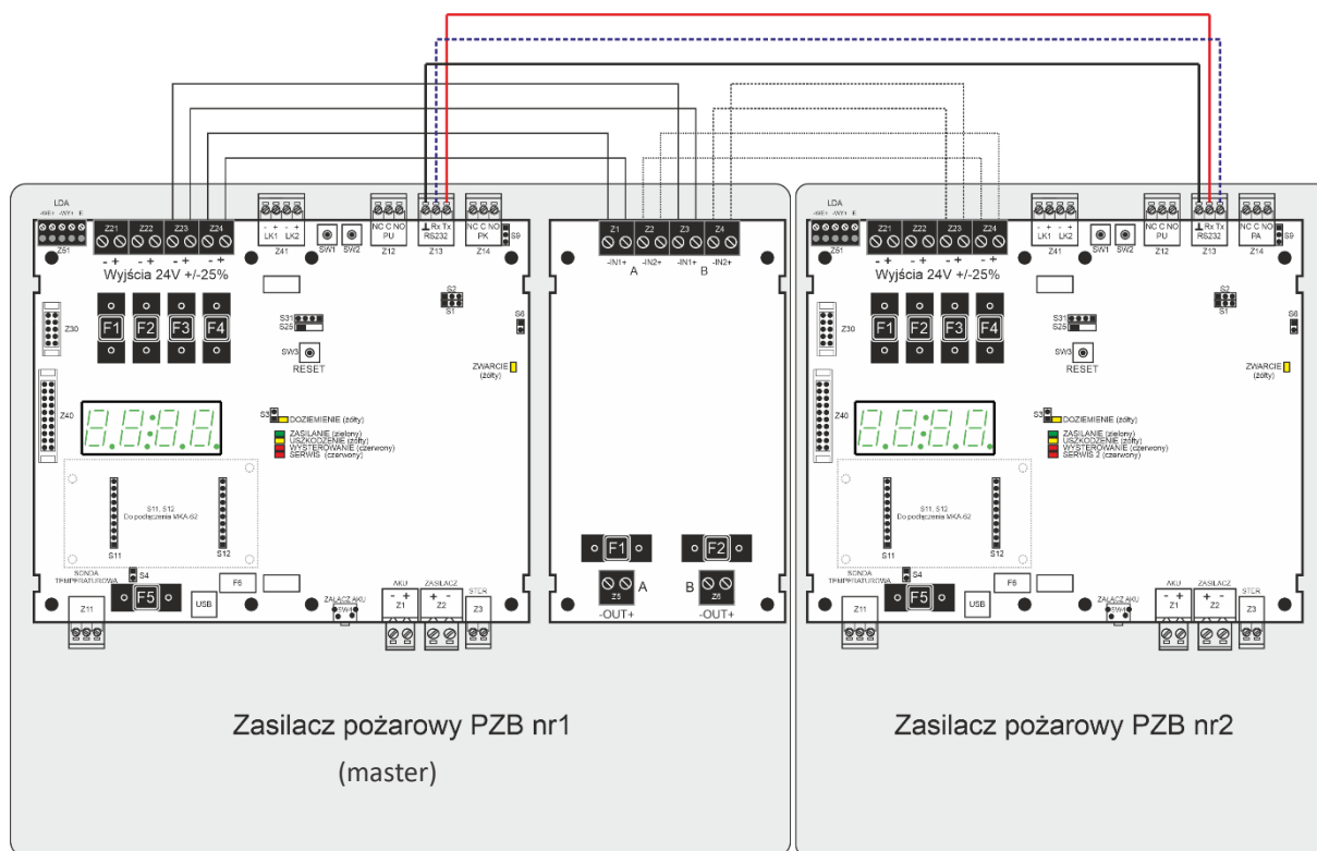
Rysunek 6.5.2. Przedstawienie połączeń modułu redundancji z dwoma zasilaczami pożarowymi
