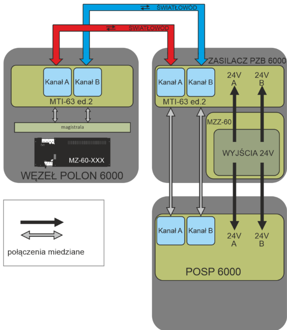
Rysunek 10.1. Schemat blokowy podłączenia POSP 6000 z centralą za pośrednictwem światłowódów i modułu MTI-63 Ed.2 zamontowanego w obudowie zasilacza PZB 6000.
