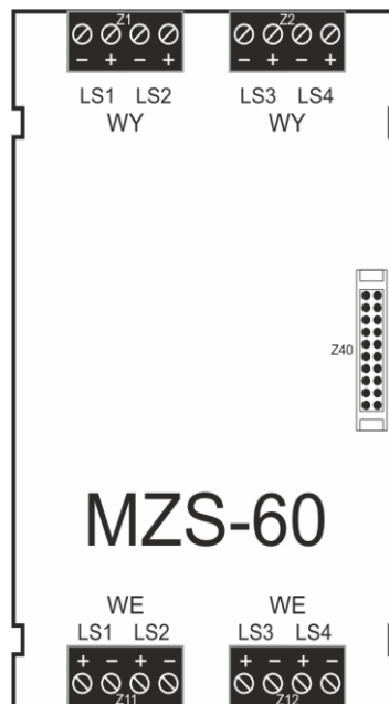
Rysunek 6.3.1. Opis wejść oraz wyjść złącza Modułu Zarządzania Sygnalizacją MZS-60
