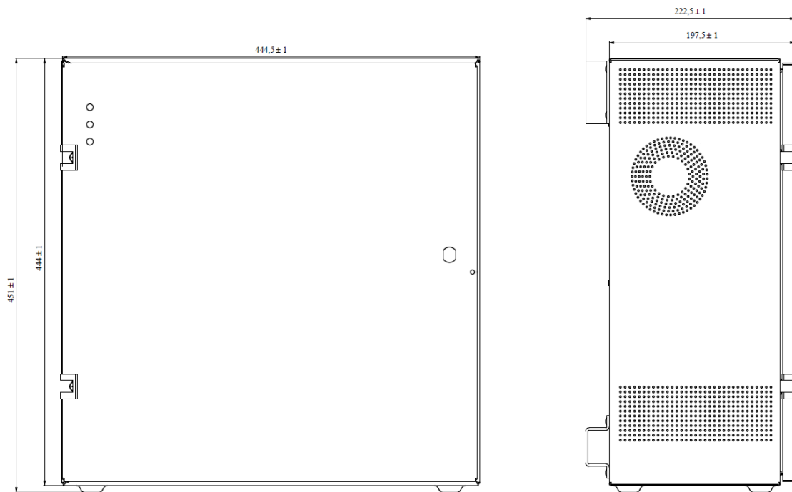
Rysunek 4.2. Obudowa M71
