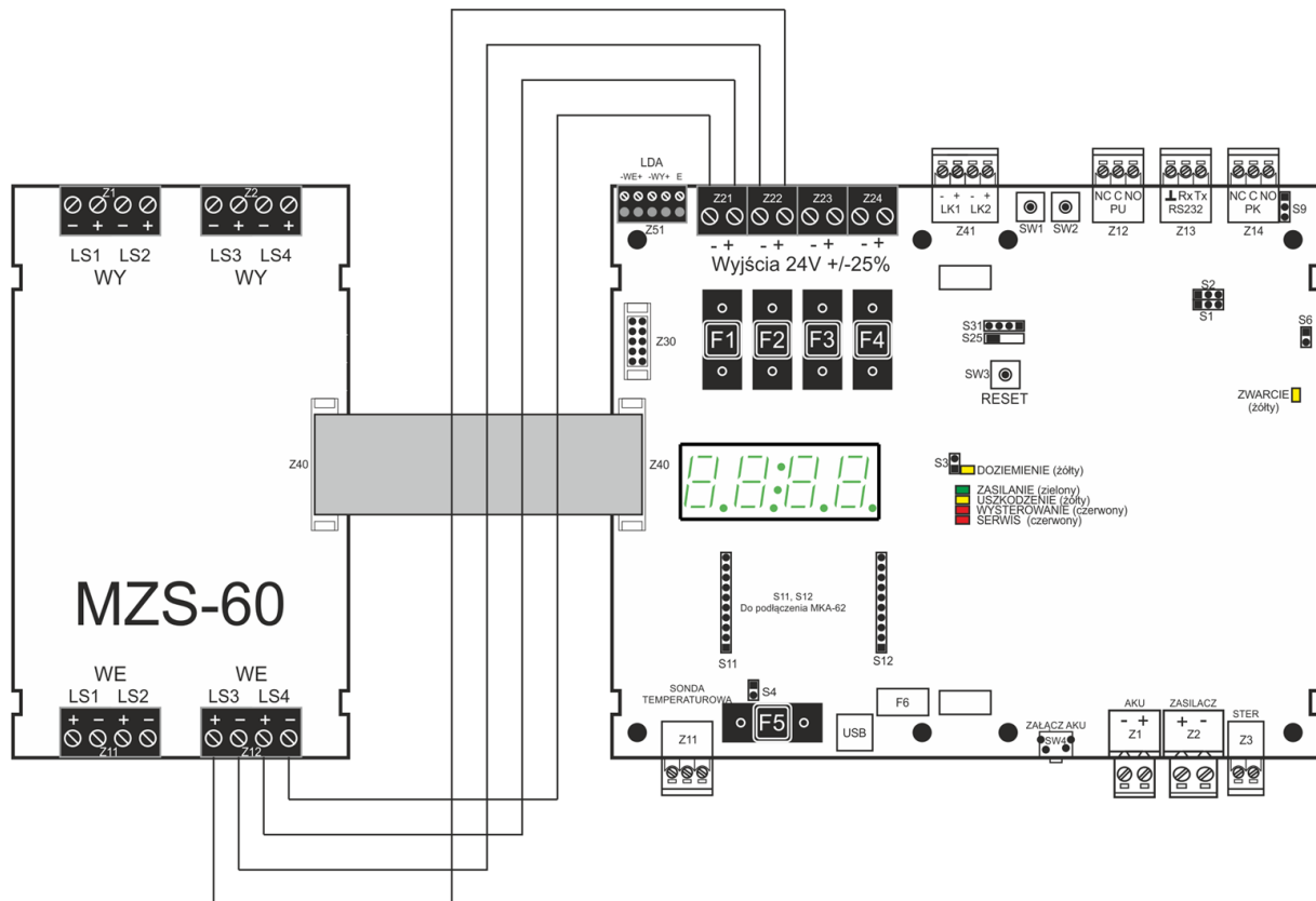
Rysunek 6.3.2. Sposób podłączenia modułu zarządzania sygnalizacją MZS-60 z modułem zarządzania zasilaniem MZZ-60
