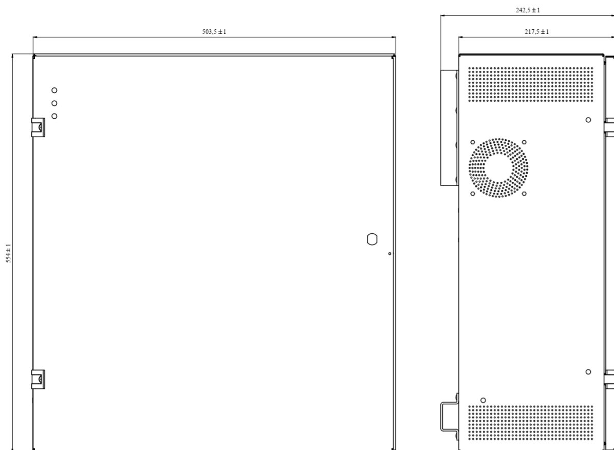
Rysunek 4.3. Obudowa M72
