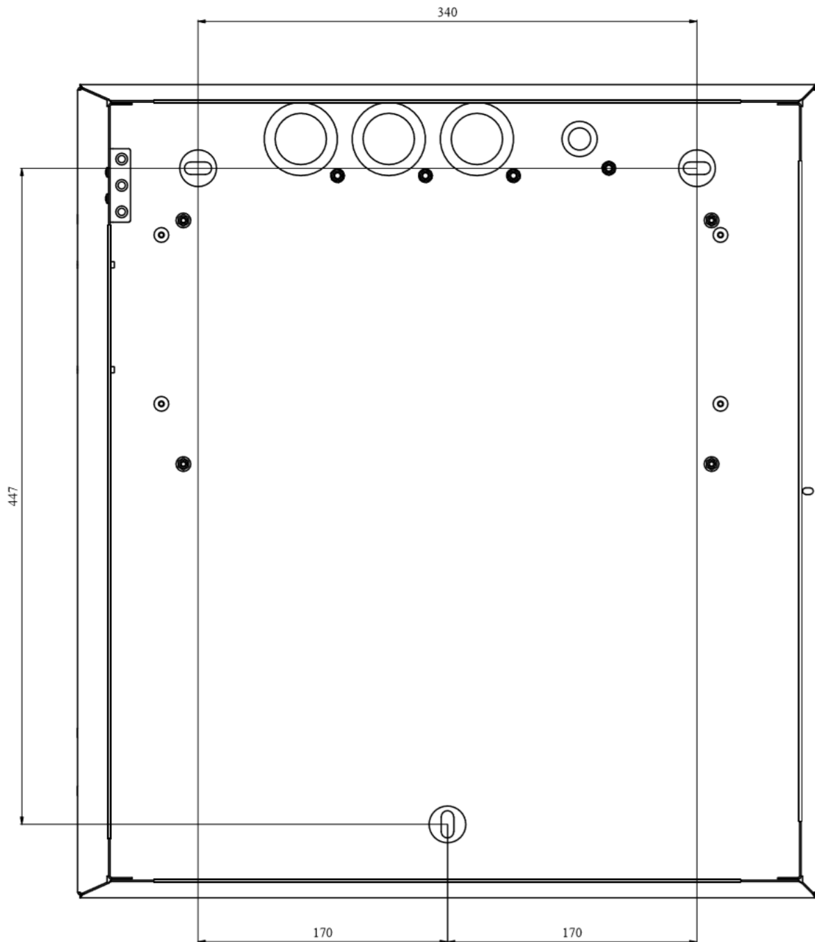
Rysunek 11.1.3. Wymiary montażowe obudowy M72
