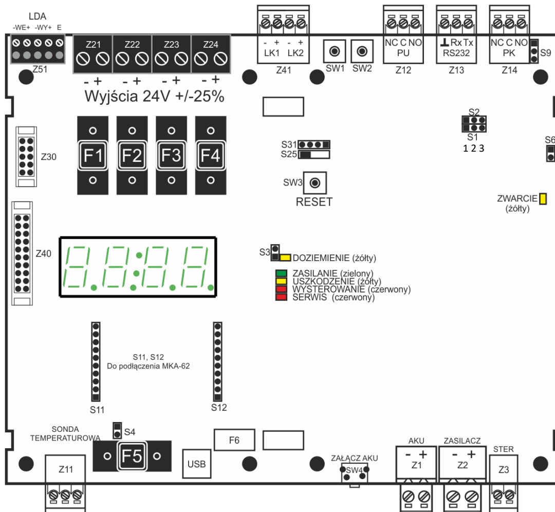
Rysunek 6.2.1. Opis wejść oraz wyjść złącz modułu MZZ-60 Pożarowego Zasilacza Buforowego
