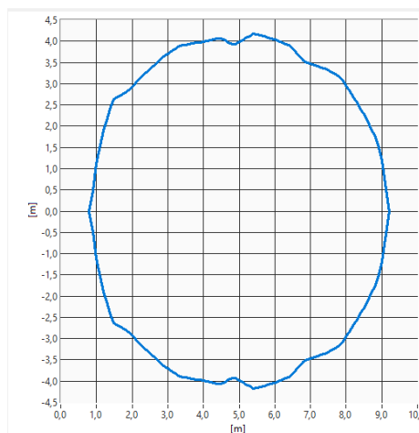
Rys. 7.2.2. Przekrój podłużny w odległości x=4 m od osi optycznej sygnalizatora SO-P8/CC, SO-P8/BC bryła 6m
