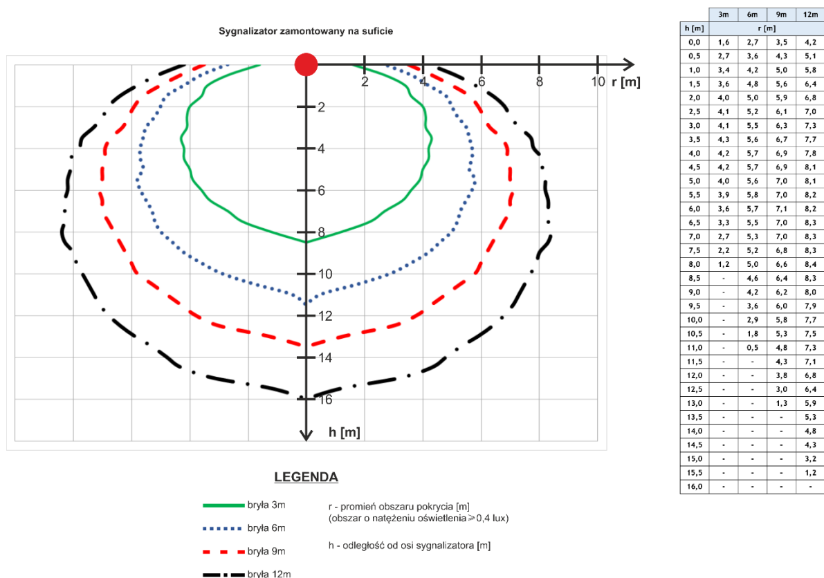
Rys. 7.2.2.1. Przekroje brył fotometrycznych w zależności od wybranej bryły sygnalizatora SO-P8/CC, SO-P8/BC oraz promień obszaru pokrycia (r) w zależności od wysokości montażu (h).
