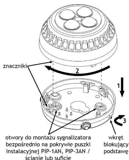
Rys. 6.1. Otwieranie / zamykanie sygnalizatora SO-P8.
