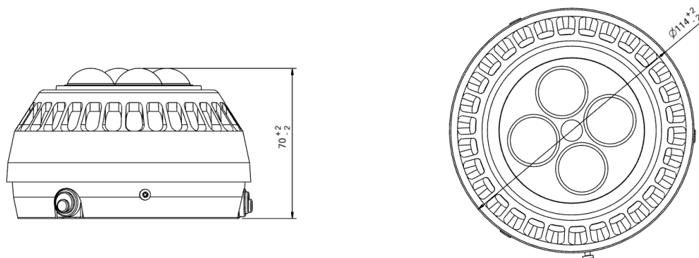
Rys 7.3.1. Wymiary sygnalizatora SO-P8.
