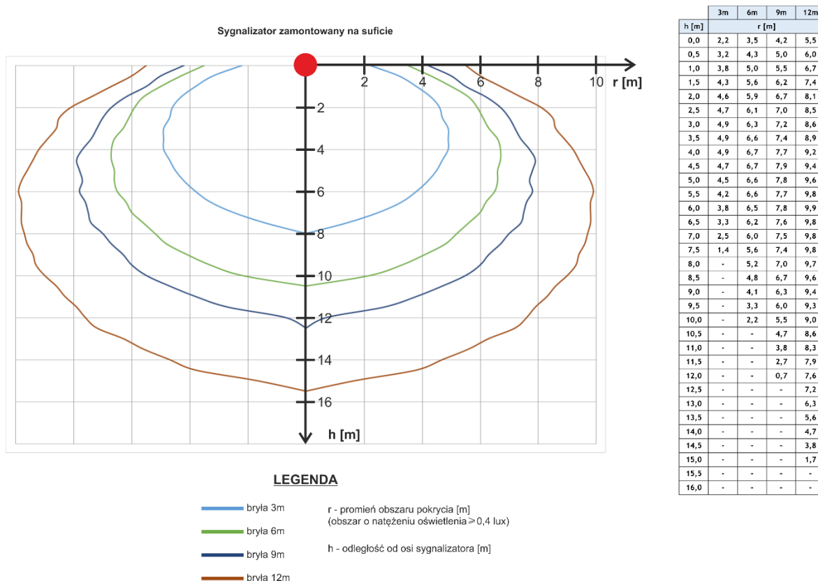
Rys. 7.2.3.1. Przekroje brył fotometrycznych w zależności od wybranej bryły sygnalizatora SO-P8/CB, SO-P8/BB oraz promień obszaru pokrycia ( r ) w zależności od wysokości montażu ( h ).
