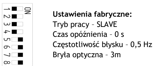
Rys. 4.3.2. Ustawienia fabryczne sygnalizatora SO-P8
