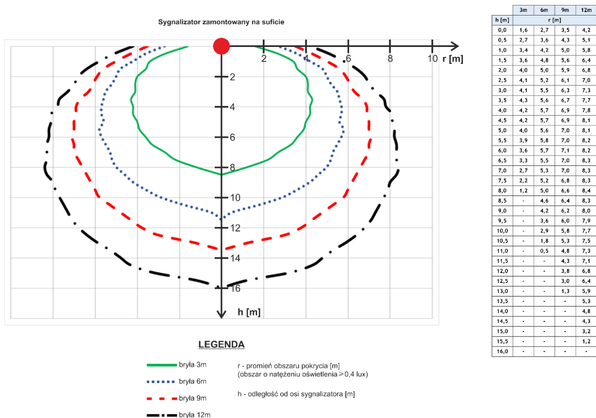
Rys. 7.3.2.1. Obszar pokrycia sygnalizatora SAO-P8/CC, SAO-P8/BC w zależności od wybranej bryły oraz wysokości montażu
