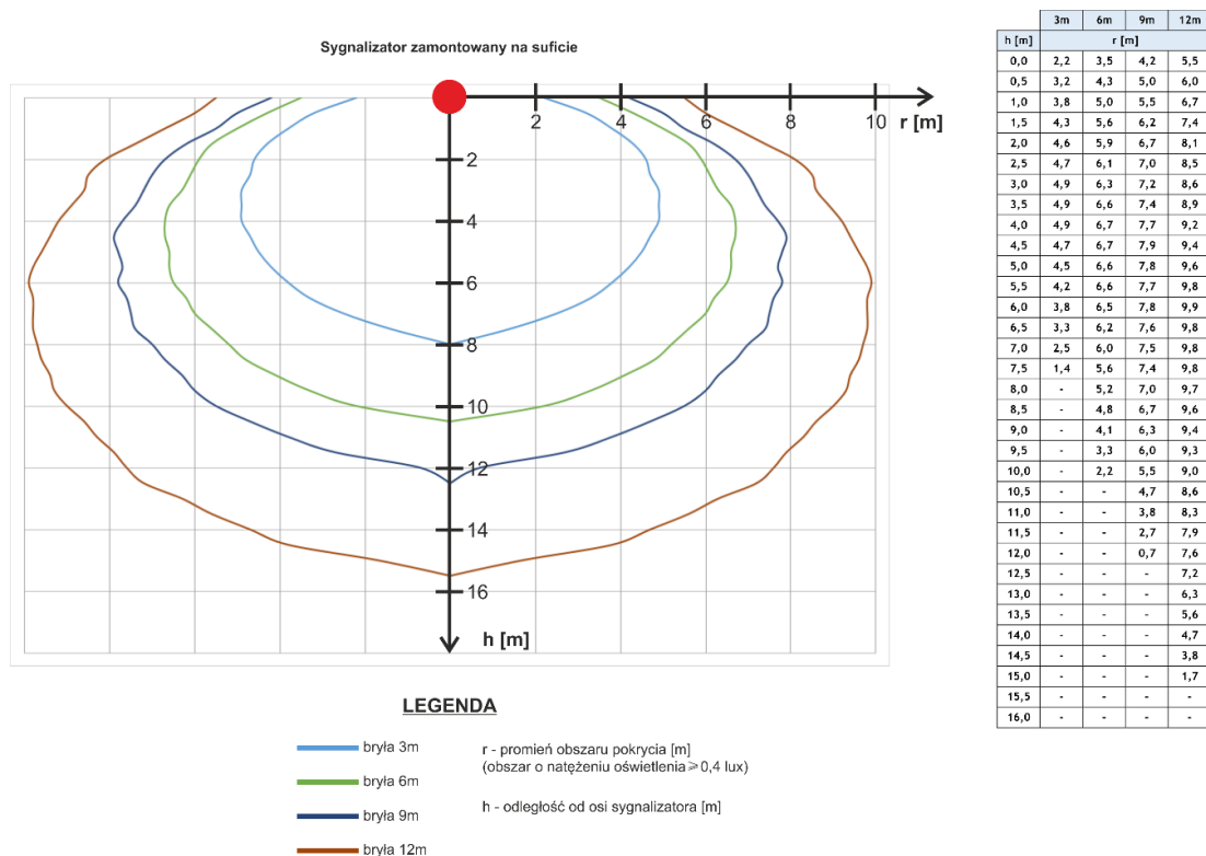
Rys. 7.3.3.1. Obszar pokrycia sygnalizatora SAO-P8/CB, SAO-P8/BB w zależności od wybranej bryły oraz wysokości montażu
