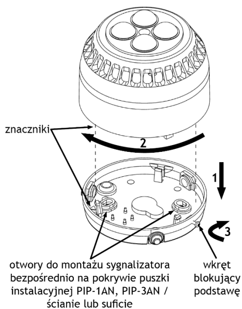
Rys 6.1. Otwieranie / zamykanie sygnalizatora SAO-P8.
