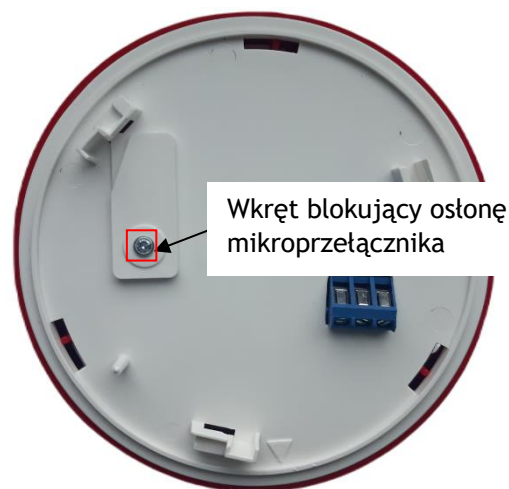
Rys. 4.3.2. Wkręt blokujący osłonę mikroprzełącznika
