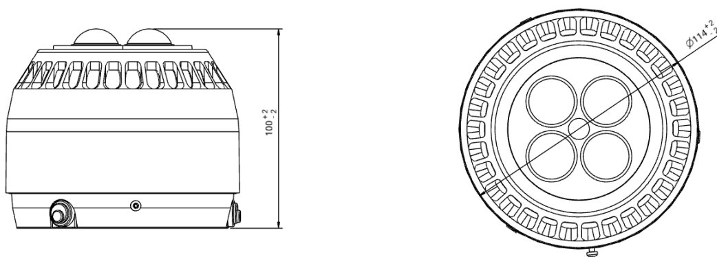
Rys. 7.4.1. Wymiary sygnalizatorów typu SAO-P8
