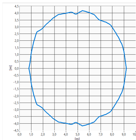
Rys. 7.3.2. Przekrój podłużny w odległości x=4 \text{ m} od osi optycznej sygnalizatora SAO-P8/CC, SAO-P8/BC bryła 6m
