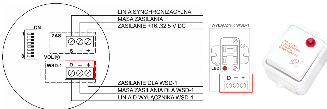
Rys. 4.5.1. Schemat podłączenia wyłącznika WSD-1 do sygnalizatora SAO-P8
