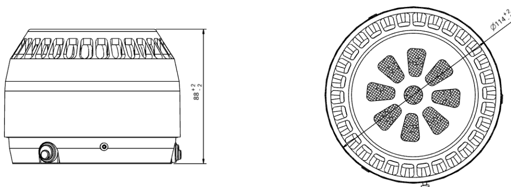
Rys. 7.4.1. Wymiary sygnalizatorów typu SA-P8
