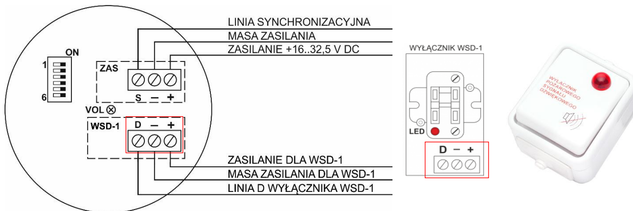
Rys. 4.5.1. Schemat podłączenia wyłącznika WSD-1 do sygnalizatora SA-P8
