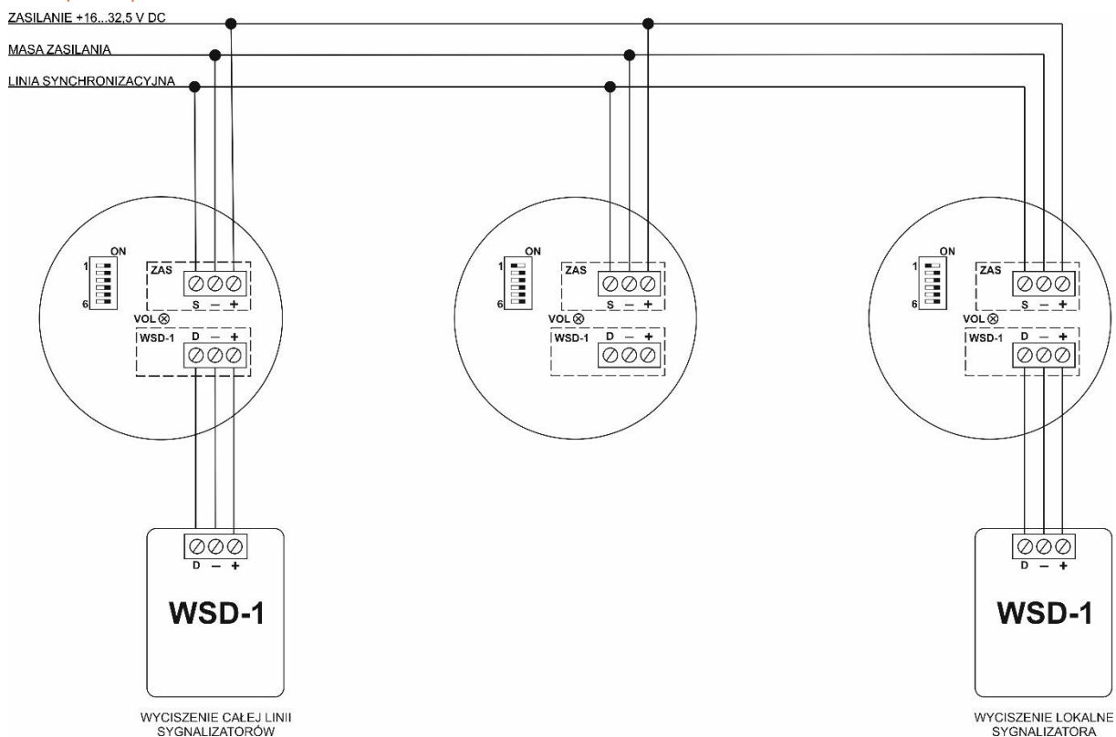
Rys. 4.4.1. Przykładowy schemat synchronizacji sygnalizatorów SA-P8
