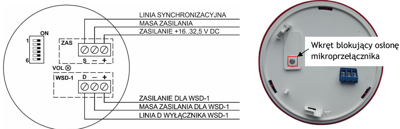
Rys. 4.3.1. Schemat podłączenia sygnalizatora SA-P8
